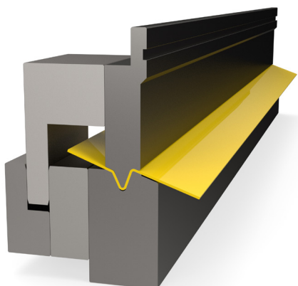
Présszerszám hátsó megvezetéssel aszimmetrikus V-kontúrhoz
