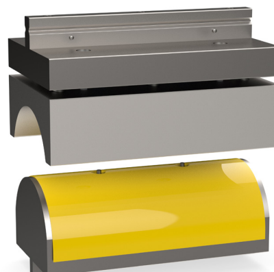
Állomás 2: Kalibráló szerzám présbéllyeggel, két benyomás egyidejű burkolatba préseléséhez
