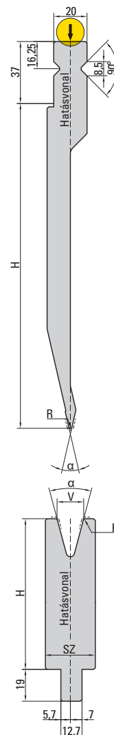
LVD Typ I.
