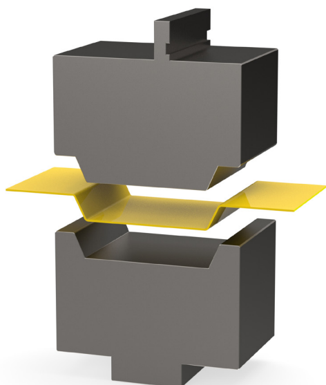
Trapézhajlító-szerszám nagy trapéz profilhoz
