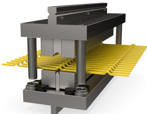
Több állomásos szerszám hullám profilok előállításához köracélból
