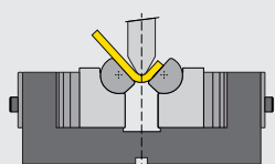
V-hajlítás
