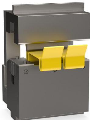
Állomás 1: U-hajlító-szerszám hátsó megvezetéssel és rugózott ledobóval
