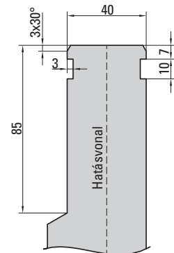
40 mm-es felfogatás
