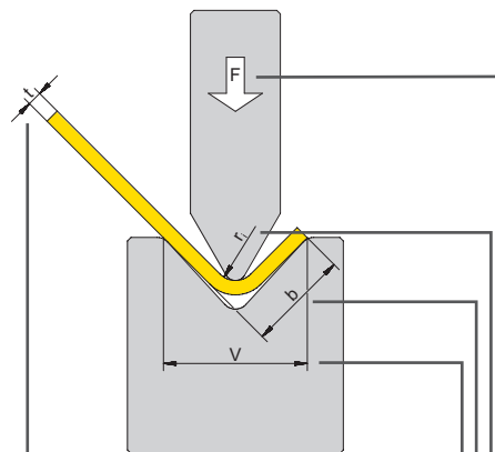
Nyomóerő-táblázat: szükséges nyomóerő 90°-os szabadon hajlításnál Szakítószilárdság R_m = 510 \text{ N/mm}^2 , acél
