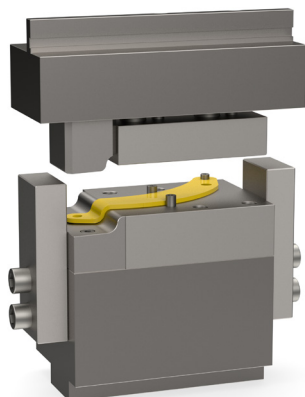
Állomás 1: Présszerszám bilincs formához, rugózott leszorítóval és oldalsó megvezetéssel
