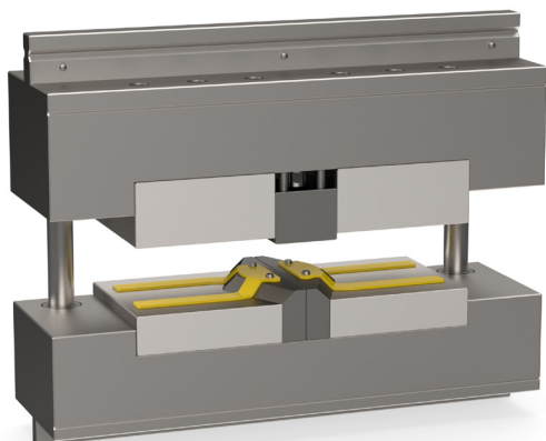
Z-présszerszám oszlopos vázzal és rugózott les- zorítással, két alkatrész löketenként
