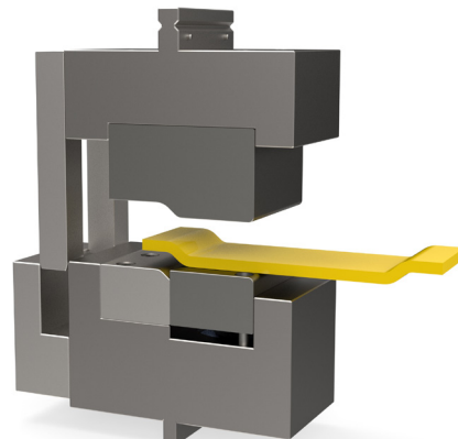
Hátsó megvezetéses Z-présszerszám
