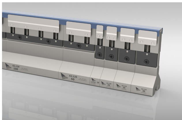
Modell 62.120 folyamatos Slider (csúszkával)
