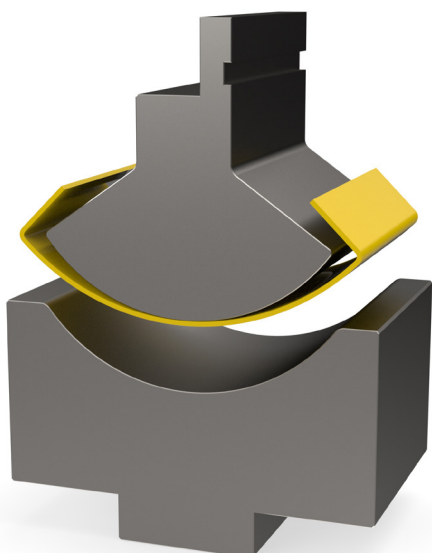
Rádiuszpréselő szerszámok nagy rádiuszokhoz, előhajlított oldalakkal
