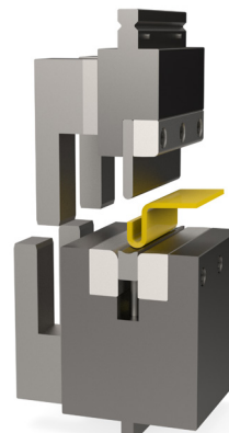
U-hajlító-szerszám hátsó megvezetéssel
