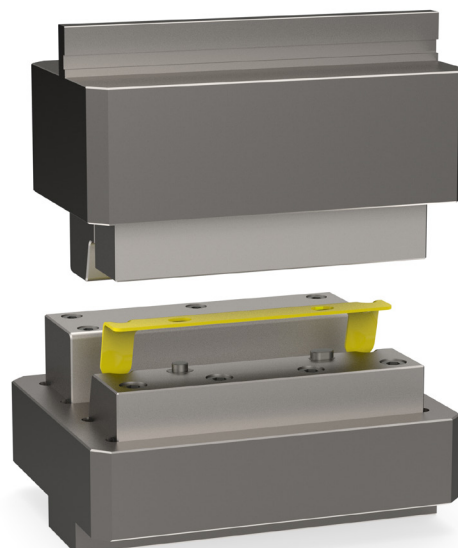
Bordanyomó-szerszám két, a hajlítási vonalhoz közel eső merevítőbordához, leszorítóval és megtámasztással, egy lökettel
