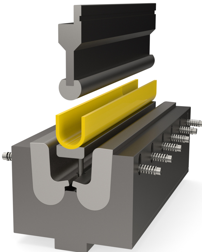
U-profil-hajlító szerszám magas felhajtással
