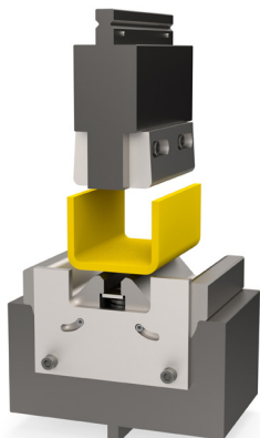
U-hajlító-szerszám beforduló pofákkal
