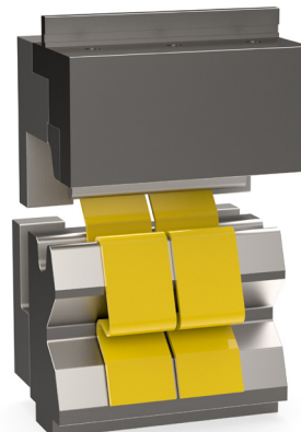
Állomás 2: Présszerszám hátsó megvezetéssel, illeszkedve az előző U-hajlító-szerszámhoz
