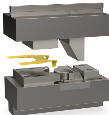
Állomás 2: Hajlító szerszám két rövid fülecske bebillentéséhez a már meghajlított szakaszokon, mozgatható éklemek segítségével
