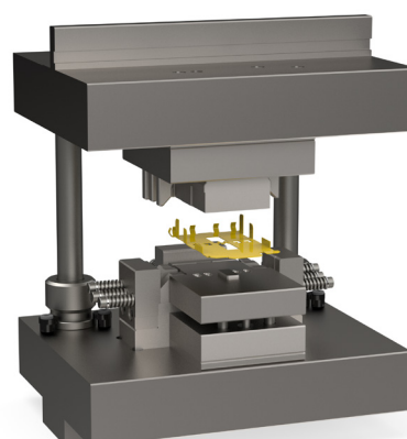
Állomás 2: több komplex kontúr készre hajlítása egy lökettel
