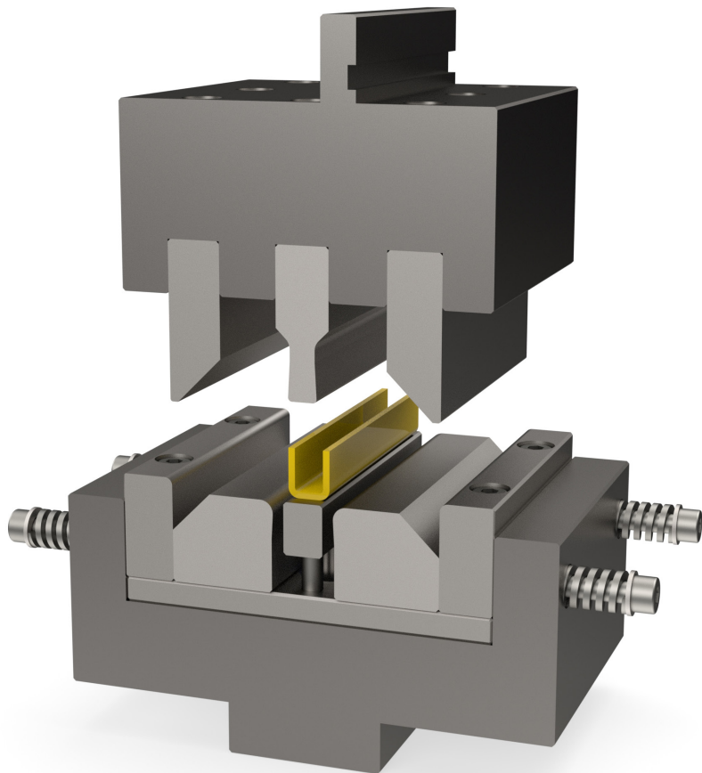
U-profil-hajlító szerszám lécceltolósos technikával az anyag visszarúgásának kompenzálására
