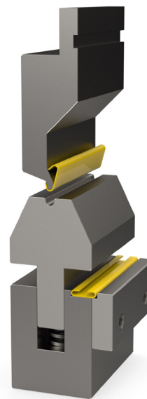
Peremező szerszámok kis C-profilhoz
