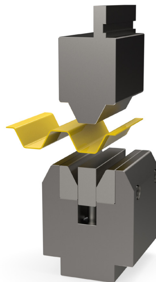
Trapézhajlító-szerszám rugózott ledobóval
