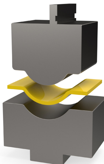
Szerszám nagy körbordákhoz
