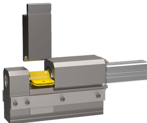
Állomás 2: csőbilincs profil zárása. Szerszám pneumatikusan vezérelt hajlítási csappal az automatizált eltávolításhoz
