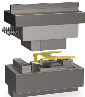
Állomás 1: Présszerszám két 90°-os hajlításhoz, 3D-kontúrral
