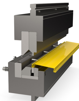
U-profil-hajlító szerszám ékeltolós technológiával és 90°-os hajlítással
