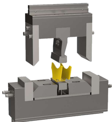
U-hajlító szerszám ékeltolások technológiával aszimmetrikus U-profilokhoz
