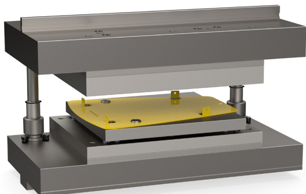
Oszlopos megvezetésű egyedi szerszám négy belső 90°-os hajlítás előállításra egy lökettel
