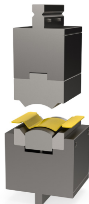
Présszerszámok hullám profilok előállítására
