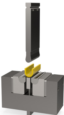
U-profil-hajlító szerszám mozgó hajlítópofákkal és ledobóval
