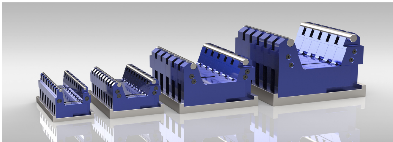
Állítható UKB-matricák 65.125, 65.185, 65.300 és 65.400
