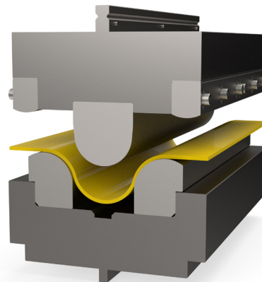
Bordanyomó szerszám állítható hajlítólécekkel
