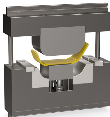
Oszlopos megvezetésű szerszám két különböző rádiusz egyidejű hajlításához
