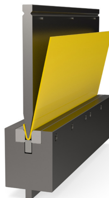
Szerszám 20°-os hajlításhoz rugózott ledobóval
