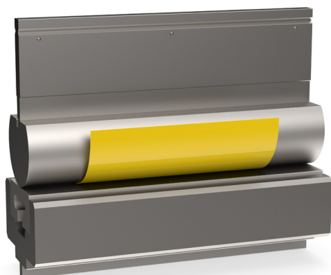
Állomás 1: Rádiuszszerzám PU-párnával lenyomatmentes, 180°-os rádiusz hajlításhoz
