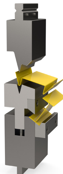
Peremező szerszámok mindkét oldali peremezésre és 90°-os hajlításra
