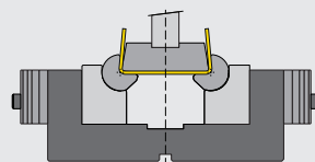
U-hajlítás
