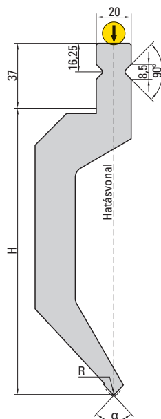
Wila Typ I.
