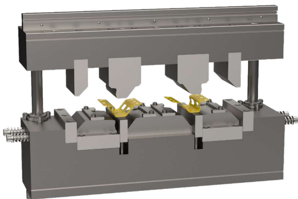
Több állomásos szerszám
