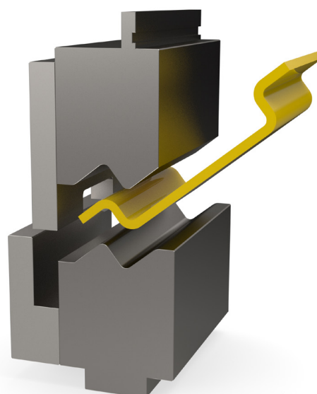
Z-hajlító-szerszám hátsó megvezetéssel, vastag anyagokhoz
