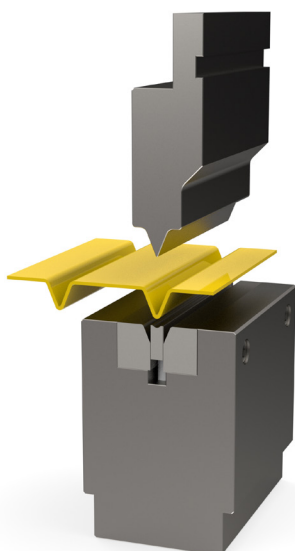
Szerszám hosszanti V-bordákhoz, rugózott ledobóval
