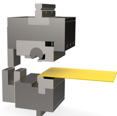
Egyedi szerszám 90°-os horizontális hajlítás előállításra
