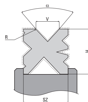
Multi-V matrica megfogatás
