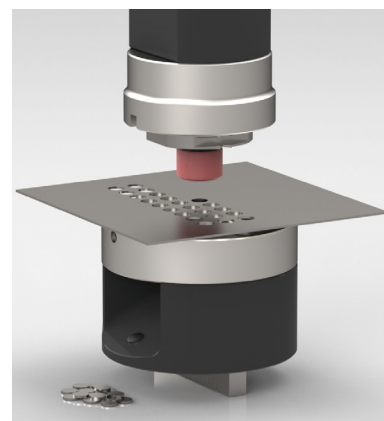
Nyílás az egyszerű hulladék eltávolításhoz és PU lehúzó lyukasztó szerszámok használata
