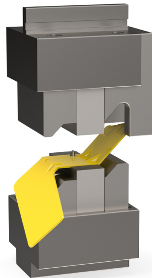
Egyedi szerszám Z-profilokhoz. Vezetett és rugózott, négy erevítőbordához, egy lökettel
