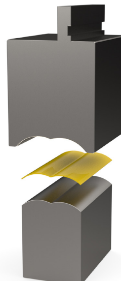
Dupla rádiuszpréselő szerszámok
