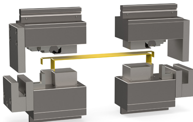
Formázószerszám rugózott leszorítóval és beforduló pofák- kal, négy 90°-os hajlítás elvégzése egy lökettel
