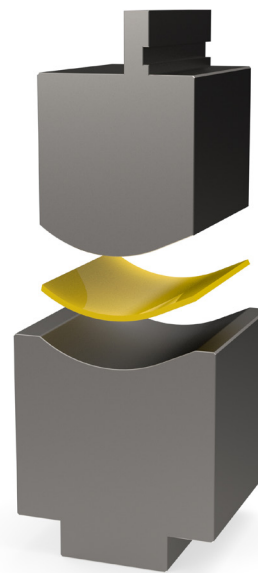
Rádiuszpréselő szerszámok egyenesen kifutó felülettel
