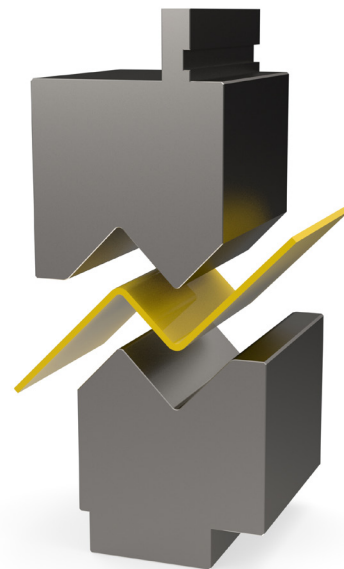
Z-hajlító-szerszám nagy lépcsőkhöz
