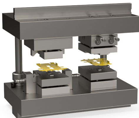
Állomás 1: különböző előhajlítások elvégzése két állomáson
