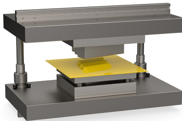
Kopolyúzó szerszám oszlopos megvezetéssel
