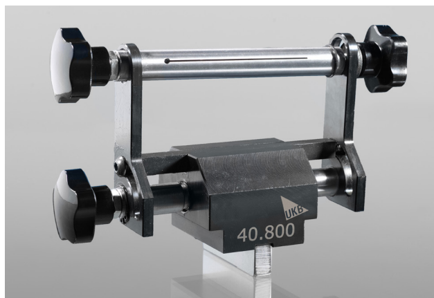
Fóliatartó tájolóléccel UKB-Trumpf/Wila/Bystronic rendszerekhez
