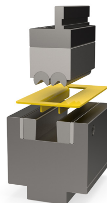
Egyedi szerszám mozgó hajlítópofákkal két belső 90°-os hajlítás előállítására egy lökettel
