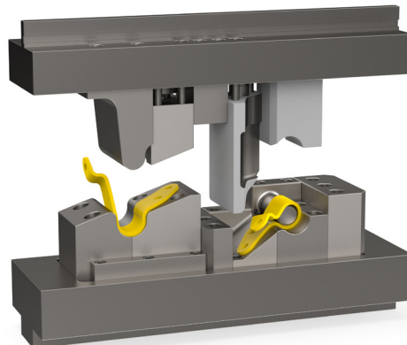
Állomás 2: Szerszám rádiusz préseléshez (bal oldal) és bilincsforma hengerítéséhez (jobb oldal), rugózott leszorítóval és beépített alátámasztással
