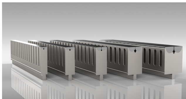
UniBend matricák 29.000, 29.100, 29.150, 29.200 és 29.300
