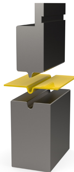
Szerszám kis körbordákhoz
